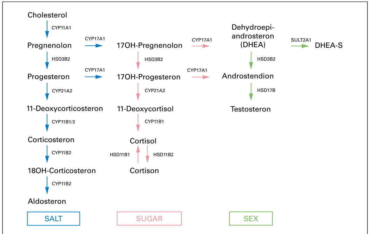
Abbildung 1: Adrenale Steroidhormonbiosynthese.
