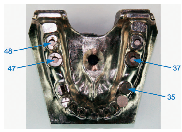
Abbildung 1 Metallguss-Standard mit den ausgewählten Markern zur Längenmessung mittels Koordinatenmessmaschine PMM 864 und Mikrotomographie.
